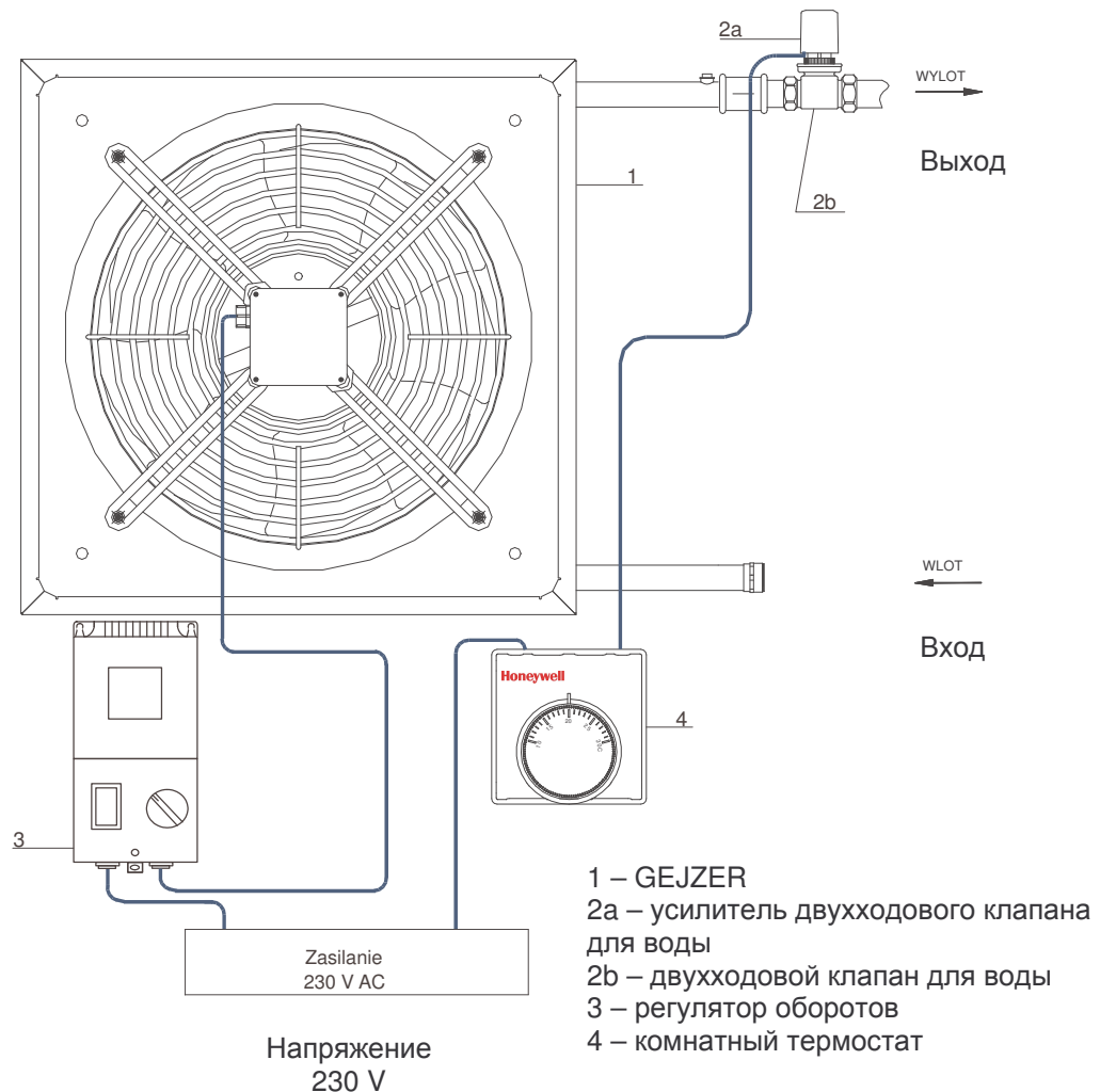
Рис. 8.1 Система управления
